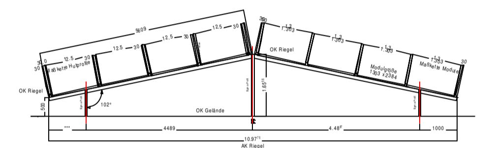
Modulschnitt Ost-West Ausrichtung M 1:100
